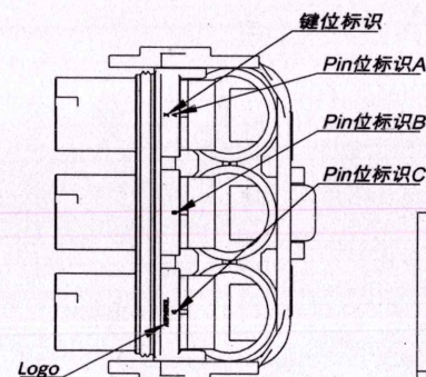
M向视图
